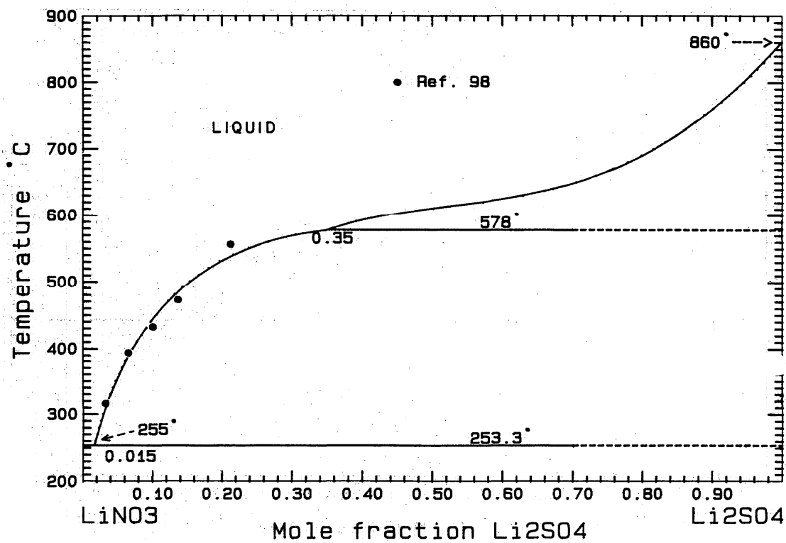
FIG. 26. The system \text{LiNO}_3 - \text{Li}_2\text{SO}_4 .
