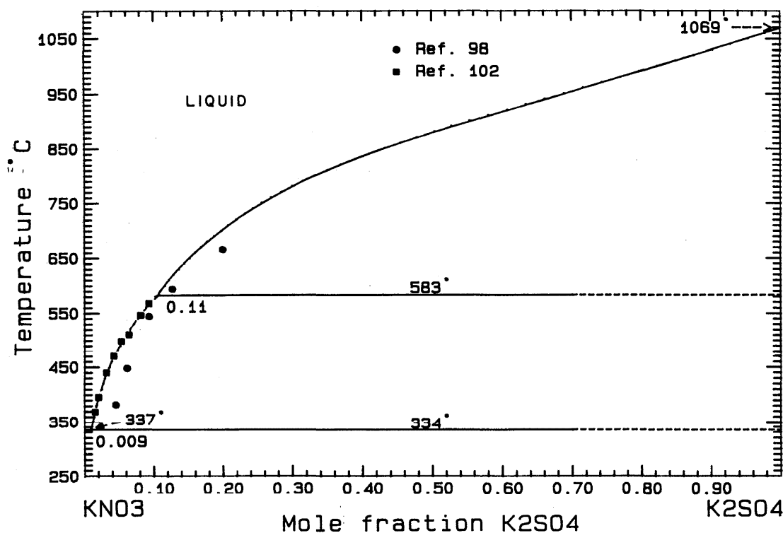
FIG. 29. The system \text{KNO}_3\text{-K}_2\text{SO}_4 .
