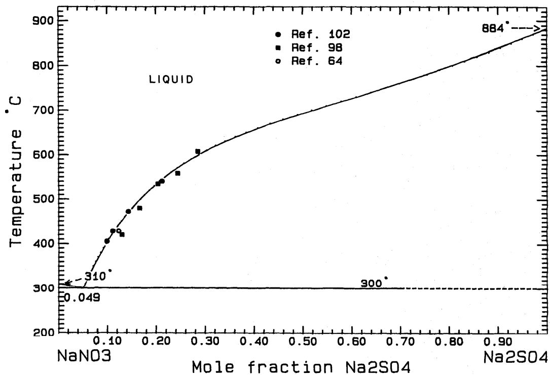
FIG. 27. The system \text{NaNO}_3 - \text{Na}_2\text{SO}_4 .
