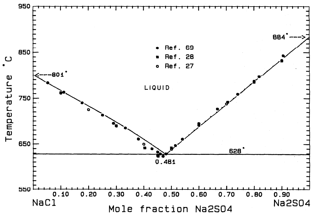
FIG. 11. The system NaCl-Na 2 SO 4 .
