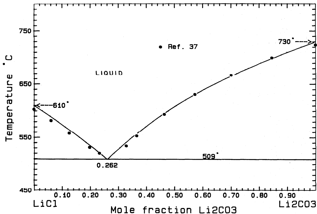
FIG. 7. The system \text{LiCl-Li}_2\text{CO}_3 .
