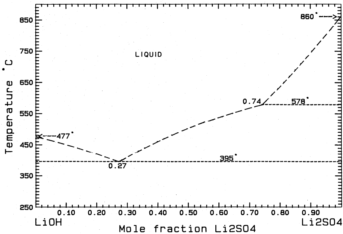
FIG. 18. The system \text{LiOH} - \text{Li}_2\text{SO}_4 .
