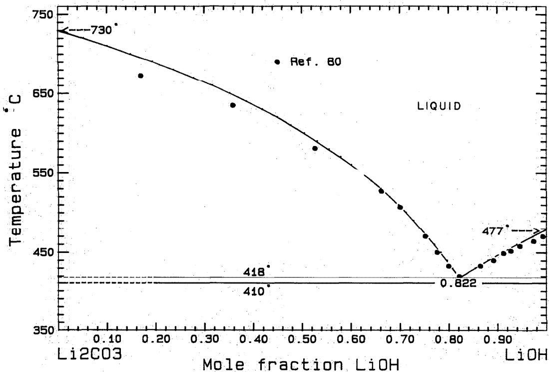
FIG. 13. The system \text{Li}_2\text{CO}_3 - \text{LiOH} .
